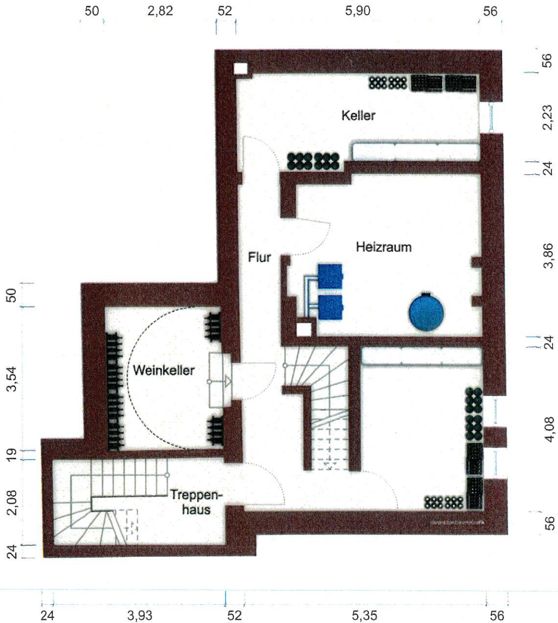
Kellergeschoss
